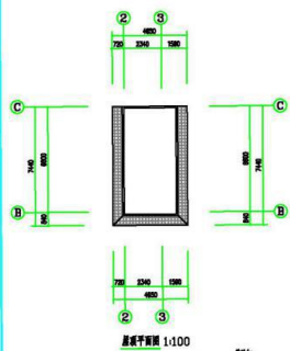
层间平面图 1:100
