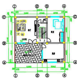
一层平面图 1:100 本层建筑面积: 102.68m 2 总建筑面积: 336.61m 2 一层庭院占地面积: 102.68m 2
