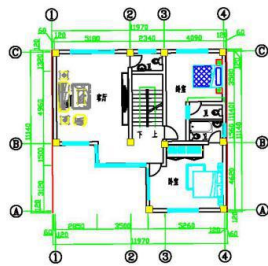
二层平面图 1:100 本层建筑面积: 107.92m 2 总建筑面积: 336.61m 2
