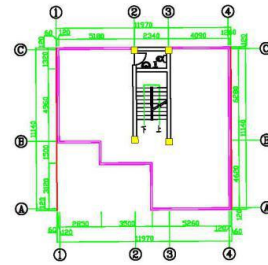
四层平面图 1:100 本层建筑面积: 18.09m 2 总建筑面积: 336.61m 2
