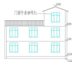
背立面图
