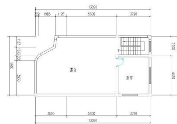
顶层平面图 顶层建筑面积: 26平方米
