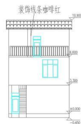
右侧立面图
