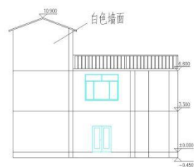
正立面图
