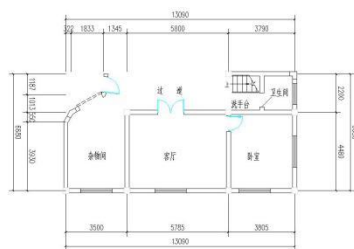
一层平面图 一层建筑面积: 86平方米
