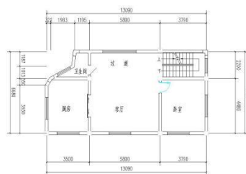
二层平面图 二层建筑面积: 86平方米
