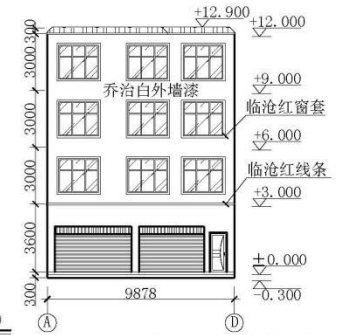
①—④轴立面图 1:300
