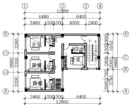
四层平面布置图 1:300 本层建筑面积: 103.39m 2
