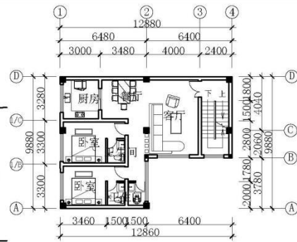
二层平面布置图 1:300 本层建筑面积: 103.39m 2
