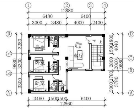
三层平面布置图 1:300 本层建筑面积: 103.39m 2
