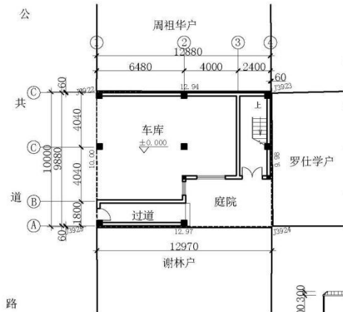
一层平面布置图 1:300 本层建筑面积: 103.39m 2
