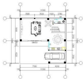
一层平面图 1:300
