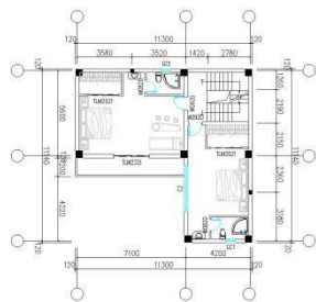
二层平面图 1:300
