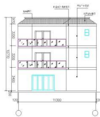
①~③立面图 1:300
