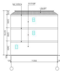
③~①立面图 1:300
