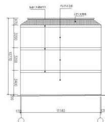
A~①立面图 1:300
