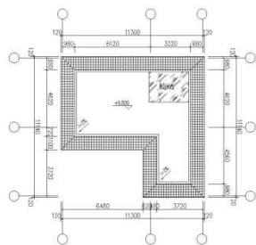
屋面平面图 1:300
