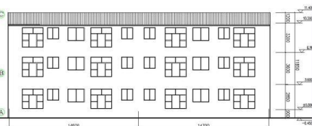
⑦~①立面图 1:100
