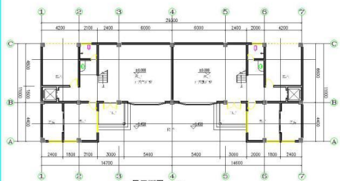
一层平面图 1:100
