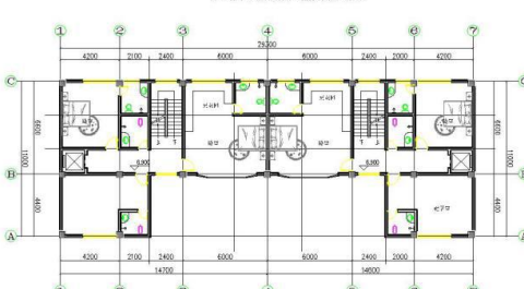
三层平面图 1:100
