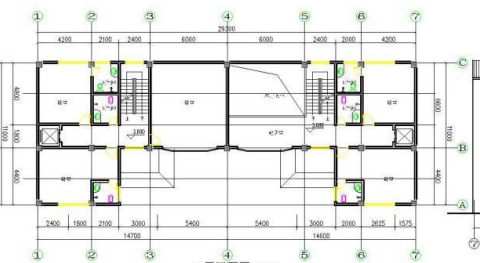
二层平面图 1:100
