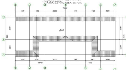
屋顶平面图 1:100
