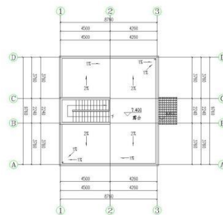
屋顶平面图 1:100
