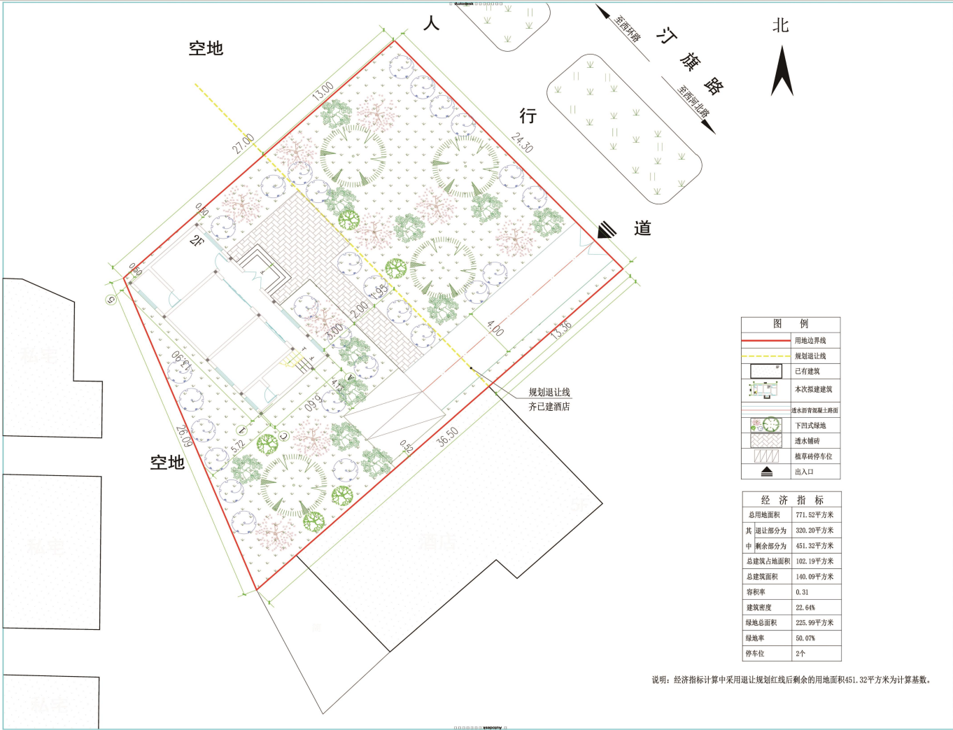
总平面布置图
