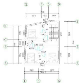
二层平面图 1:100
