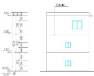
正立面 1:100
