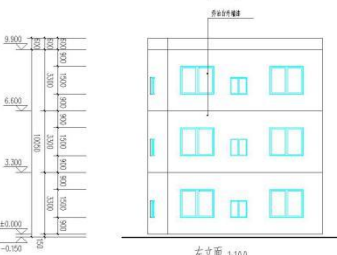
左立面 1:100
