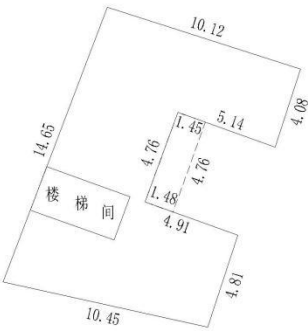
一幢三层平面图
