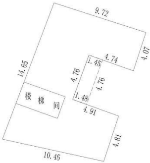
一幢一层平面图
