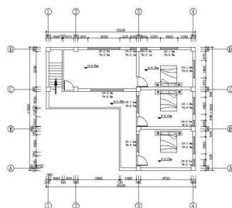
三层平面布置图 (注: 三层层高: 4m) 1:75 三层建筑面积: 98.15 \text{m}^2
