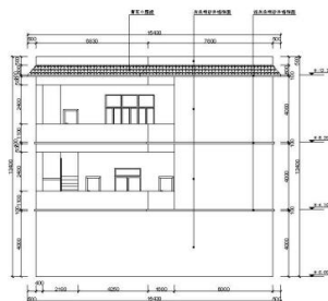
⑥-④ 建筑右立面图 占地面积: 186.67 \text{m}^2 1:75
