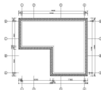
屋顶平面布置图 (注: 屋顶层高: 4m) 1:75 屋顶面积: 147.28 \text{m}^2
