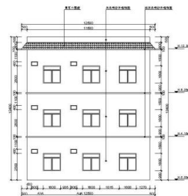
⑥-⑤ 建筑背立面图 占地面积: 186.67 \text{m}^2 1:75
