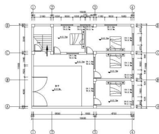
一层平面布置图 (注: 一层层高: 4m) 1:75 一层建筑面积: 98.15 \text{m}^2
