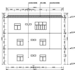
⑥-① 建筑左立面图 占地面积: 186.67 \text{m}^2 1:75
