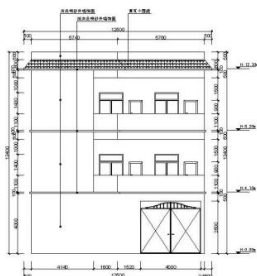
⑥-③ 建筑正立面图 占地面积: 186.67 \text{m}^2 1:75
