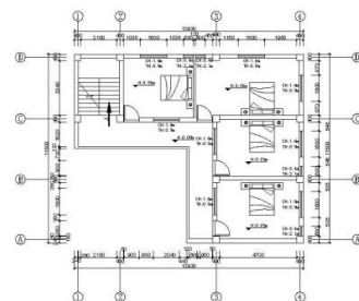
二层平面布置图 (注: 二层层高: 4m) 1:75 二层建筑面积: 96.15 \text{m}^2
