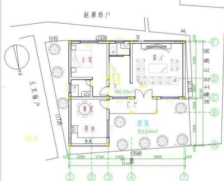
一层平面图 1:100
