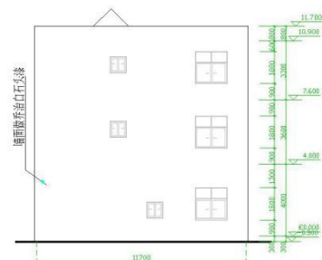
背立面图 1:100
