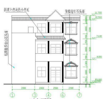
正立面图 1:100
