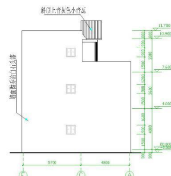
左侧立面图 1:100
