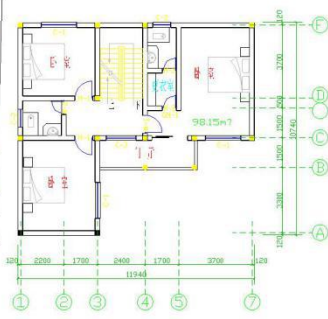
二层平面图 1:100
