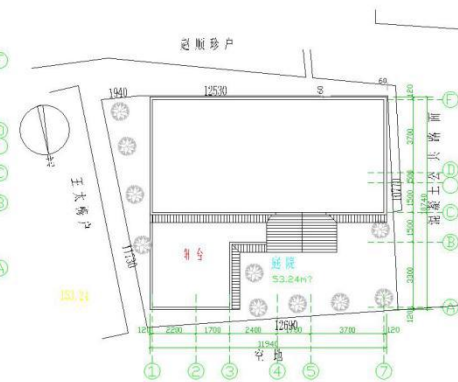
屋顶投影总平面图 1:100
