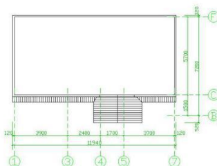
屋顶平面图 1:100
