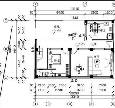
一层平面布置图: 200 本层建筑面积: 103.81m 2
