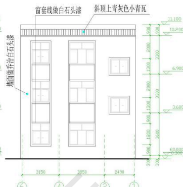
背立面图 1:100
