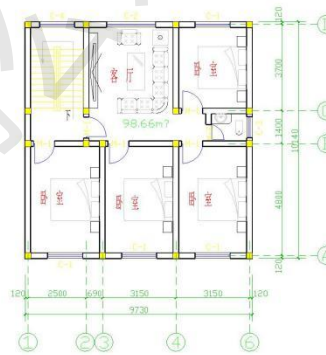
三层平面图 1:100
