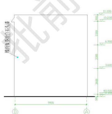
左侧立面图 1:100
