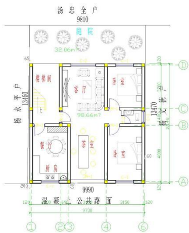
一层平面图 1:100
