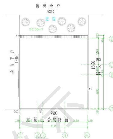
屋顶投影总平面图 1:100
