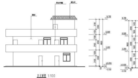
正立面图 1:100
