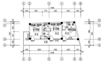
二层平面图 1:100 二层建筑面积: 67.82平方米
