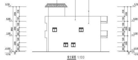
背立面图 1:100
