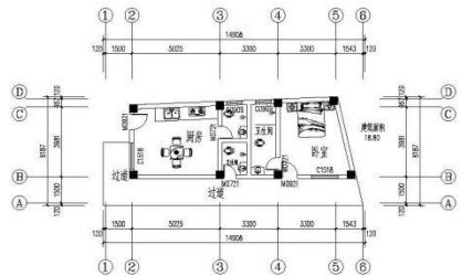
一层平面图 1:100 一层建筑面积: 67.82平方米 总建筑面积: 158.04平方米
