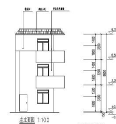
左立面图 1:100
