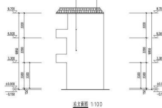
右立面图 1:100
