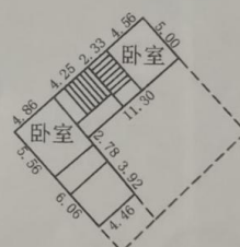
1幢2层平面图
