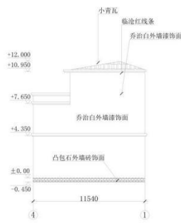
1—4 轴立面图 1:200
