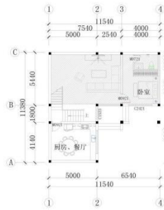
隔层平面布置图 1:200
