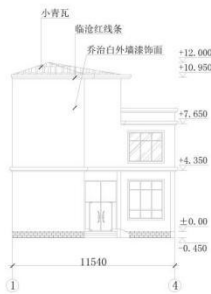
1—4 轴立面图 1:200
