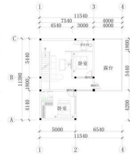
三层平面布置图 1:200
