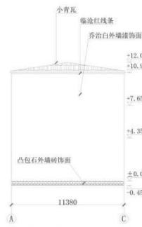
A—C 轴立面图 1:200
