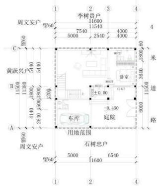
总平面图 1:200
