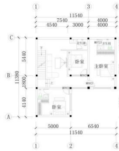
二层平面布置图 1:200
