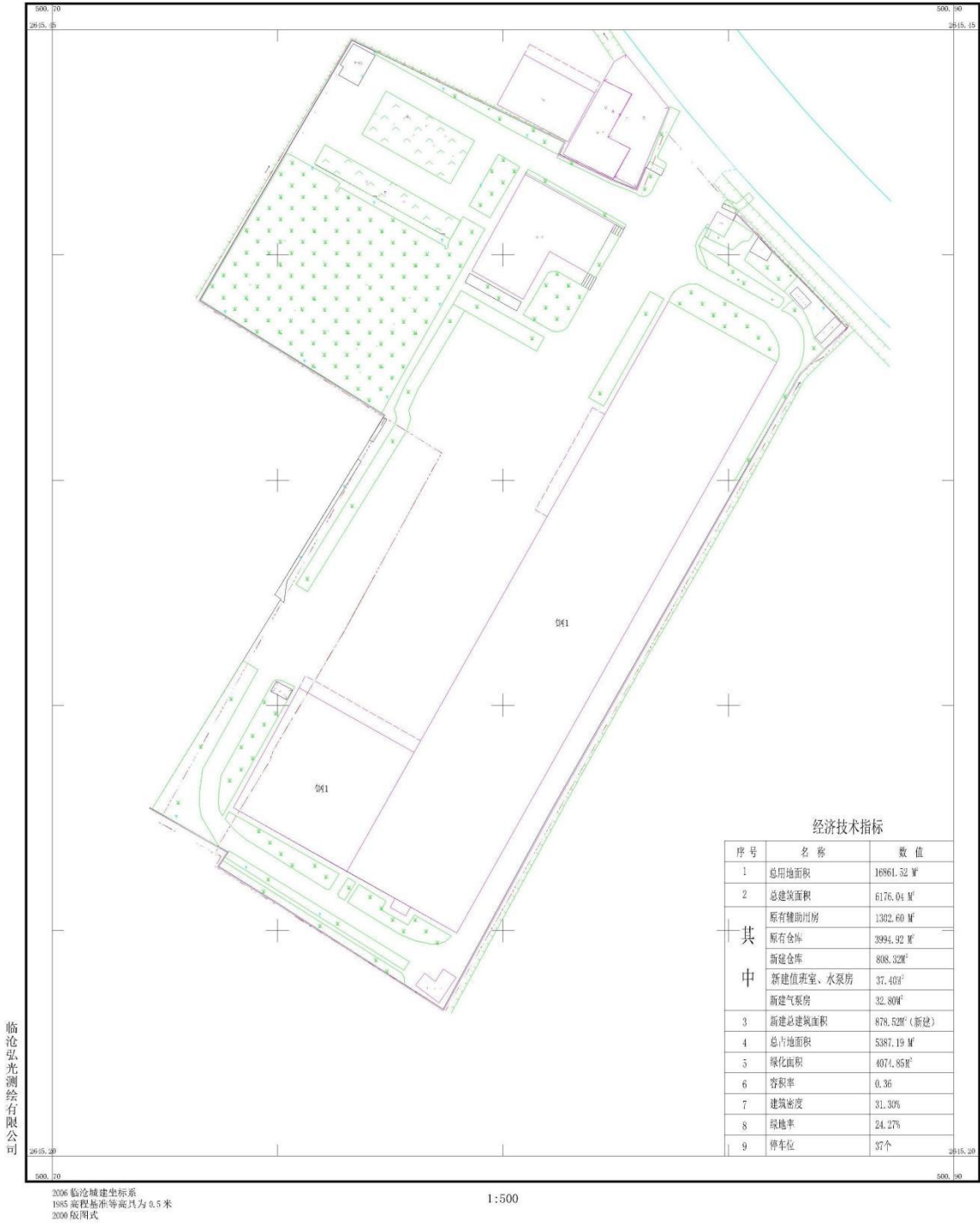
卷烟物流配送中心物料仓库新建项目竣工验收平面图 2645.200-500.700
