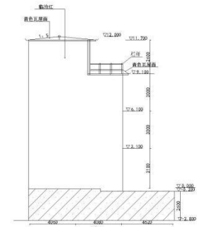
右侧面图
