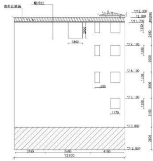
背立面图
