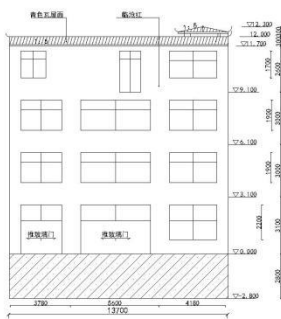
正立面图
