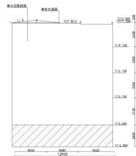
左侧面图
