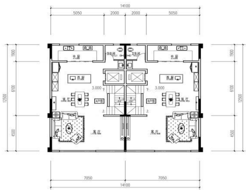
一层平面图 1:100
