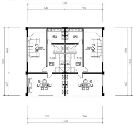
负一层平面图 1:100
