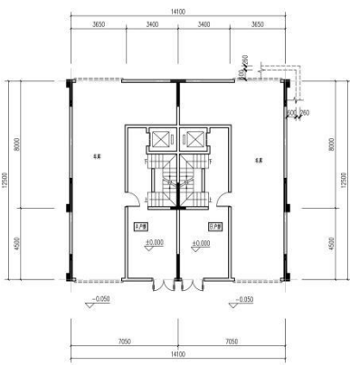
车库层平面图 1:100
