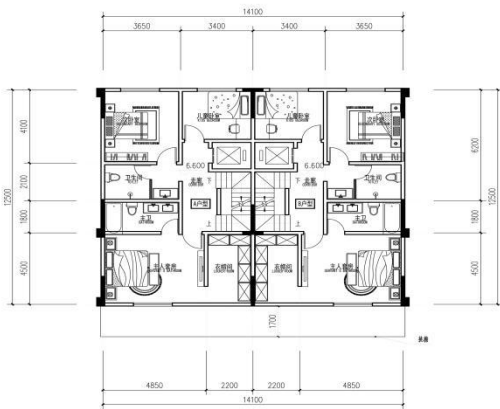
二层平面图 1:100
