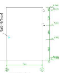
左侧立面图 1:100
