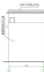
右侧立面图 1:100
