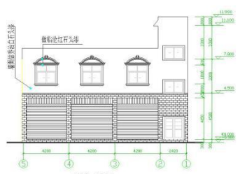
背立面图 1:100
