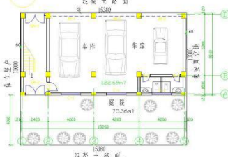
一层平面图 1:100
