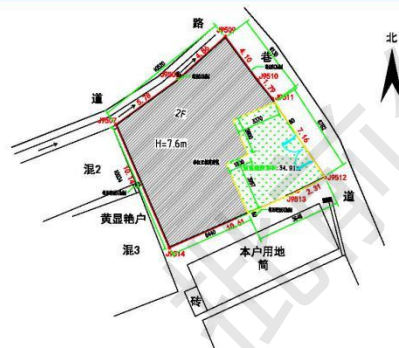
总平面布置图 1:100
