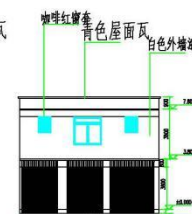
建筑南立面图 1:100
