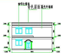
建筑正立面图 1:100
