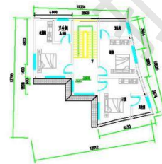
新建二层平面图 1:100
