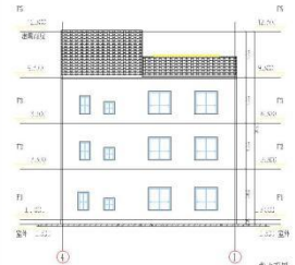
前立面图
