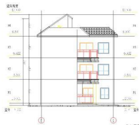
侧立面图
