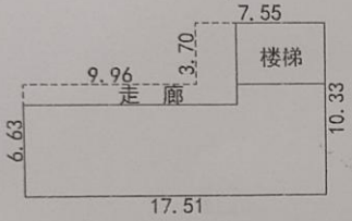
4层平面图
