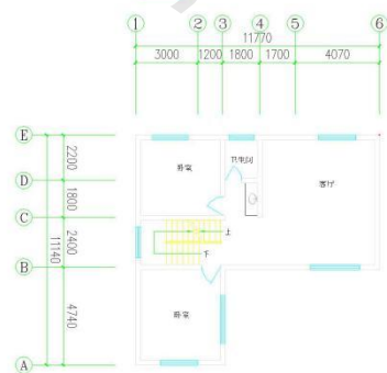
一层平面图 1:100
