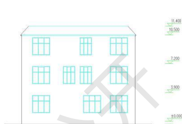
侧立面图 1:100
