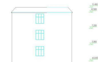
背立面图 1:100
