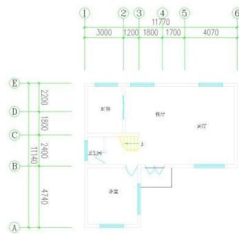
二层平面图 1:100
