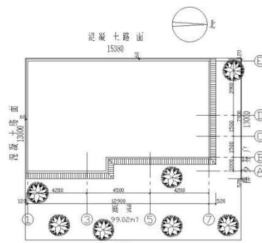
屋顶平面图 1:100
