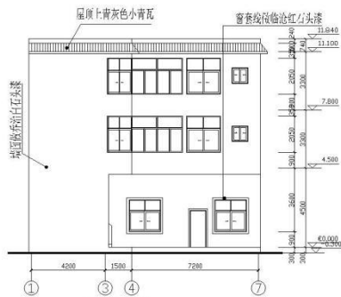
正立面图 1:100
