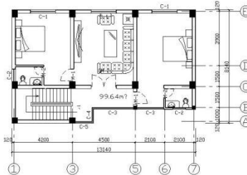
三层平面图 1:100
