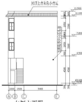
右侧立面图 1:100
