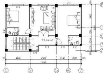
二层平面图 1:100
