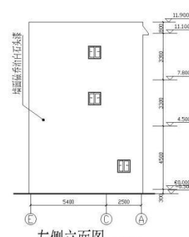
左侧立面图 1:100
