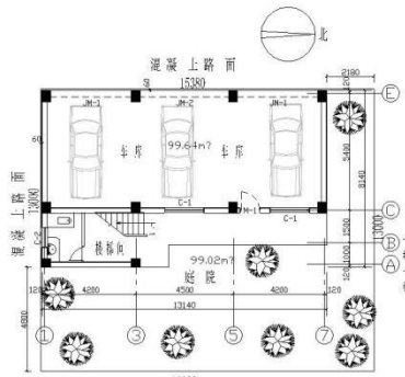
一层平面图 1:100
