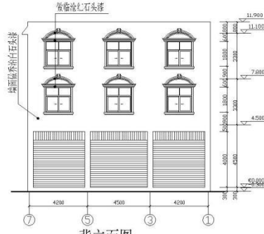
背立面图 1:100
