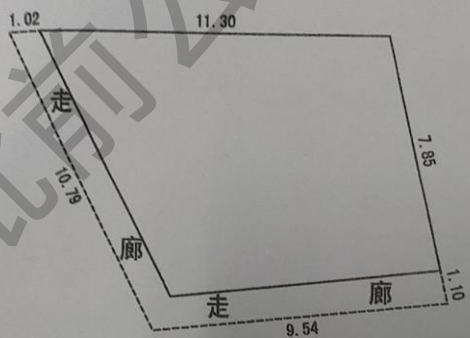
一层平面图
