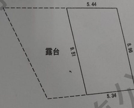
四层平面图
