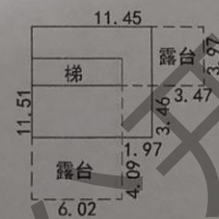
4层平面图
