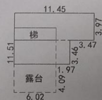
3层平面图
