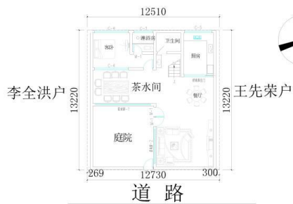
一层平面图
