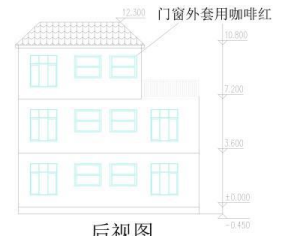
后视图
