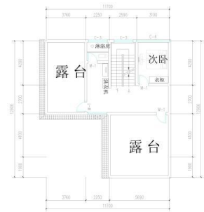
三层平面图
