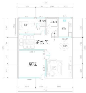
一层平面图
