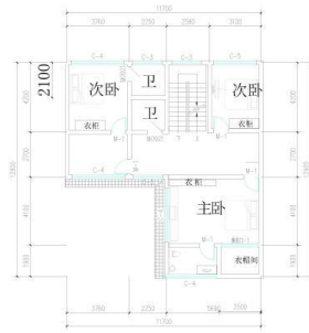
二层平面图
