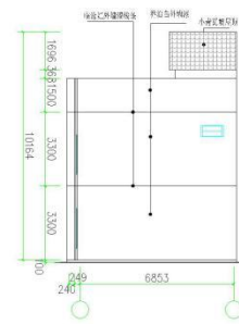
A~B立面图 1:200
