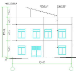
①~③立面图 1:200
