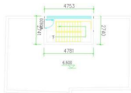
三层平面图 1:200 建筑面积: 13.05m²
