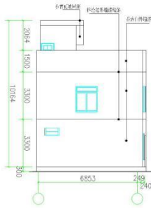
B~A立面图 1:200
