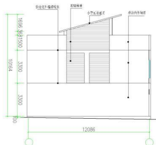
③~①立面图 1:200
