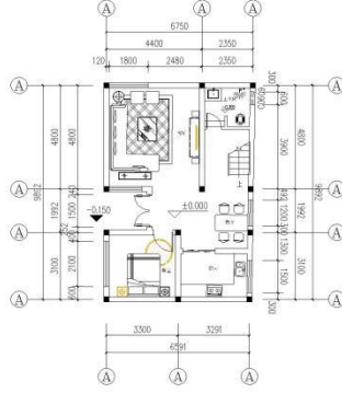
住宅2-层平面布置图 1:100
