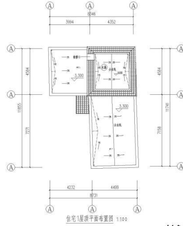
住宅1层平面布置图 1:100
