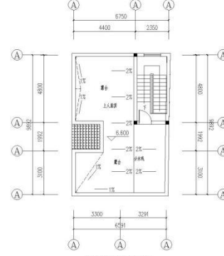
住宅2-层平面布置图 1:100
