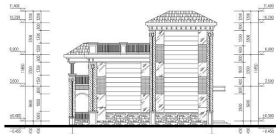
①-③轴立面图 1:100
