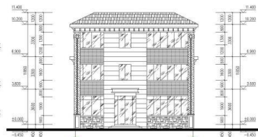
①-③轴立面图 1:100
