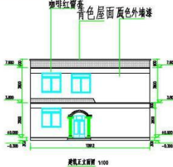
建筑正立面图 1:100
