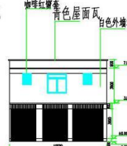
建筑南立面图 1:100
