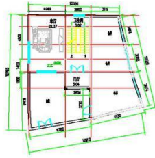
新建一层平面图 1:100 一层建筑面积: 98.18平方米
