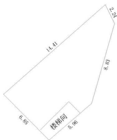
二层平面图
