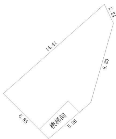
一层平面图
