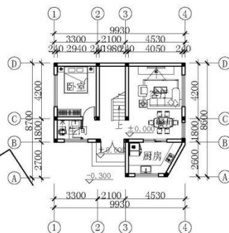
一层平面布置图1:200
