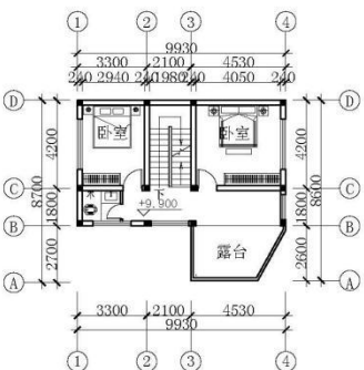
三层平面布置图1:200
