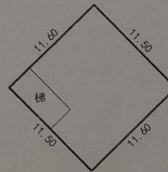
一幢一层平面图
