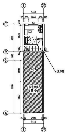
三层平面图 1:200
