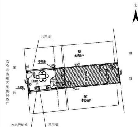
总平面布置图 1:200
