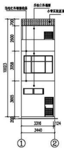
①~②立面图 1:200
