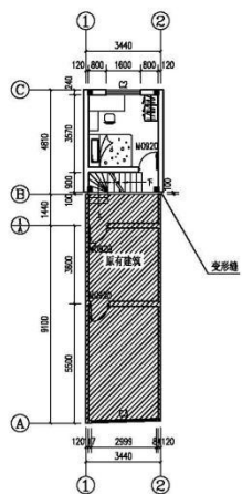
二层平面图 1:200
