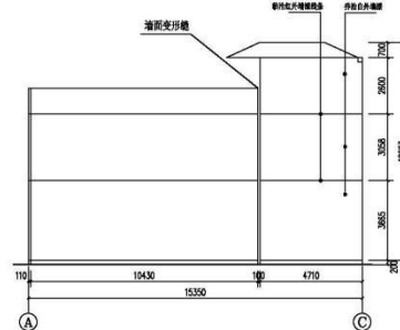
④~③立面图 1:200
