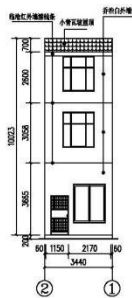
②~①立面图 1:200
