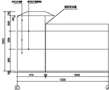
③~④立面图 1:200
