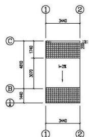
屋面平面图 1:200
