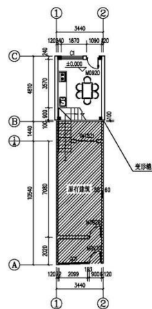
一层平面图 1:200
