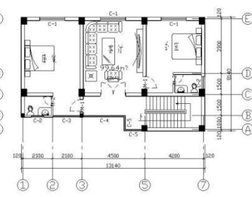
三层平面图 1:100
