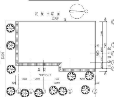
屋顶平面图 1:100
