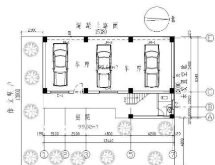
一层平面图 1:100
