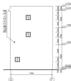
右侧立面图 1:100
