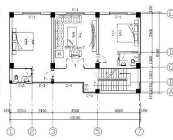
二层平面图 1:100
