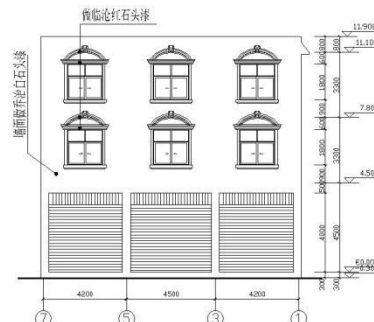
背立面图 1:100
