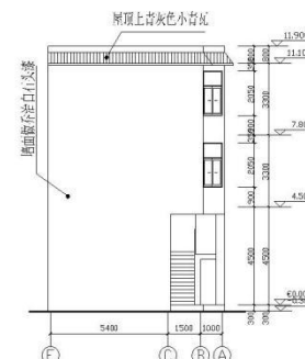
左侧立面图 1:100
