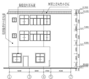
正立面图 1:100
