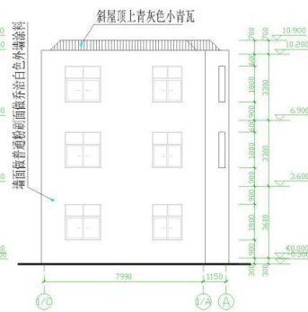
左侧立面图 1:100
