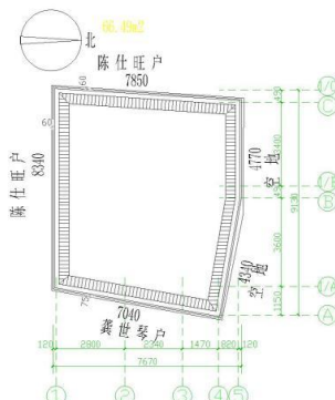
屋顶平面图 1:100
