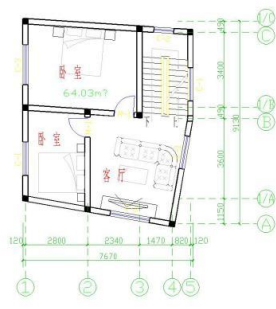
二层平面图 1:100
