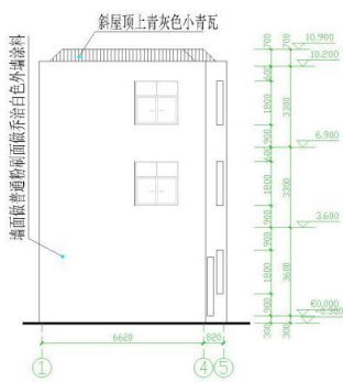
正立面图 1:100
