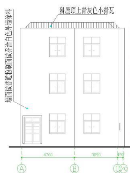
右侧立面图 1:100
