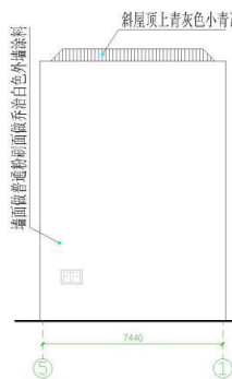
背立面图 1:100
