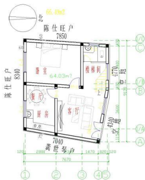
一层平面图 1:100
