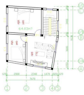
三层平面图 1:100
