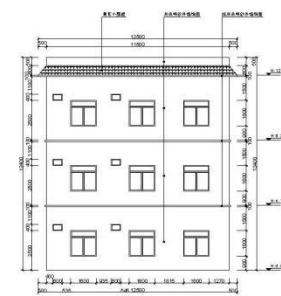
④-④ 建筑背立面图 占地面积: 188.67m 2 1:75
