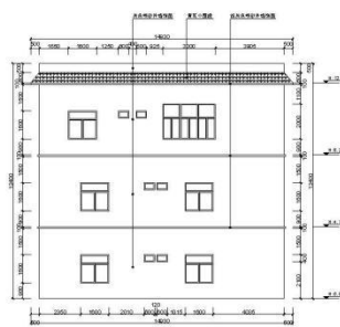
④-① 建筑左立面图 占地面积: 188.67m 2 1:75
