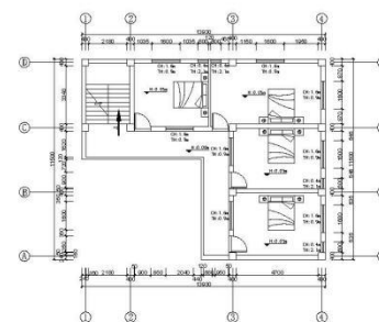
二层平面布置图 (注: 二层层高: 4m) 1:75 二层建筑面积: 98.15m 2
