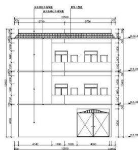
①-① 建筑正立面图 占地面积: 188.67m 2 1:75
