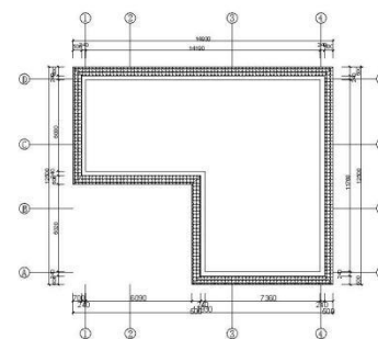
屋顶平面布置图 (注: 屋顶层高: 4m) 1:75 屋顶面积: 147.28m 2
