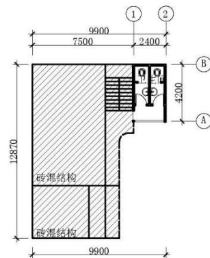
二层平面图 1:200
