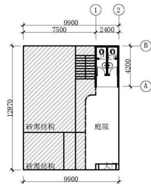
一层平面图 1:200
