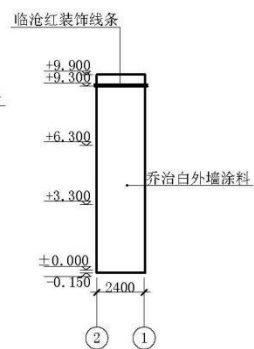
②—①轴立面图 1:200
