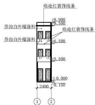
①—②轴立面图 1:200
