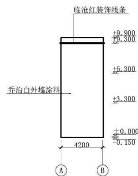
①—②轴立面图 1:200
