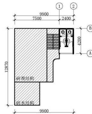
二层平面图 1:200
