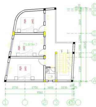
二层平面图 1:100
