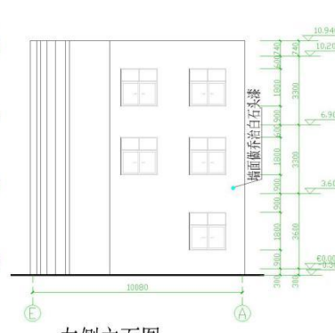
左侧立面图 1:100
