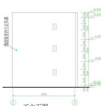
正立面图 1:100
