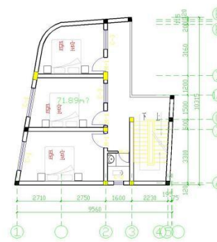
三层平面图 1:100
