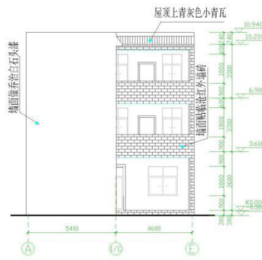
右侧立面图 1:100
