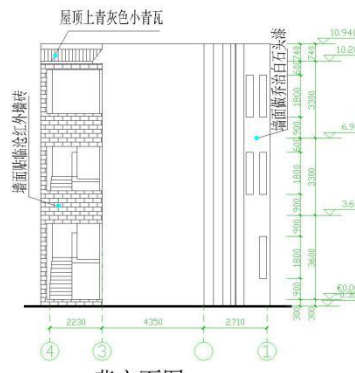
背立面图 1:100
