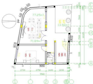
一层平面图 1:100
