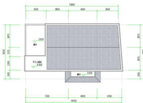
屋顶平面图 1:100
