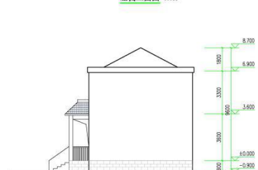
右侧立面图 1:100
