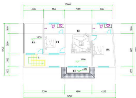
二层平面图 1:100 本层建筑面积为131.67平方米
