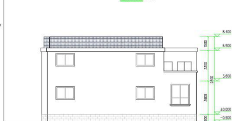
背立面图 1:100
