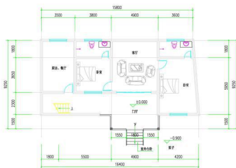
一层平面图 1:100 本层建筑面积为124.13平方米
