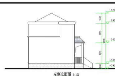
左侧立面图 1:100
