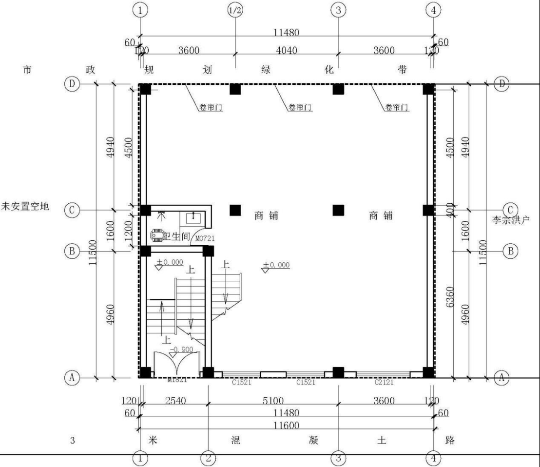
一层平面布置图1:100
