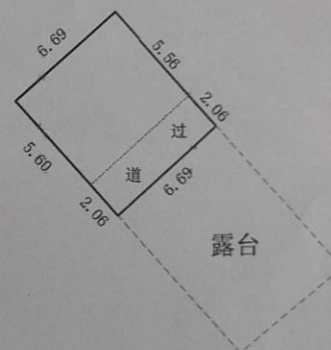
一幢三层平面图
