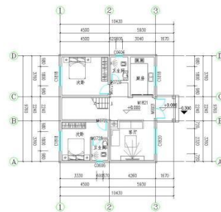
一层平面布置图 1:100 本层建筑面积 94.21平方米 建筑总面积 199.9平方米
