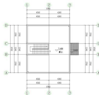
三层平面布置图 1:100 本层建筑面积 11.45平方米 建筑总面积 199.9平方米
