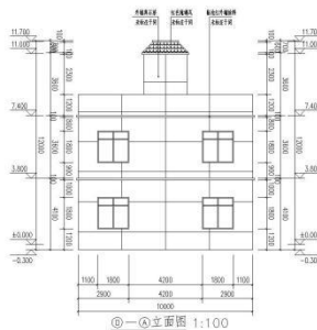
②—④立面图 1:100
