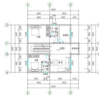
二层平面布置图 1:100 本层建筑面积 94.21平方米 建筑总面积 199.9平方米
