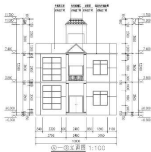
①—③立面图 1:100
