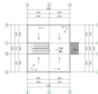
屋顶平面图 1:100
