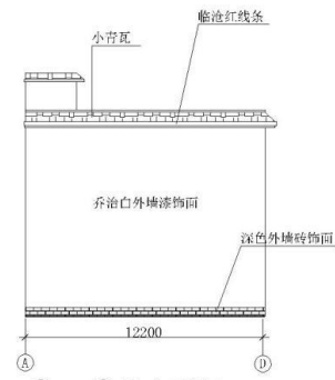
④—①轴立面图 1:200
