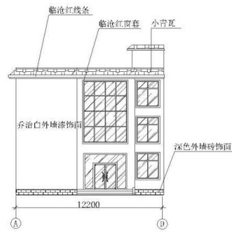
①—④轴立面图 1:200
