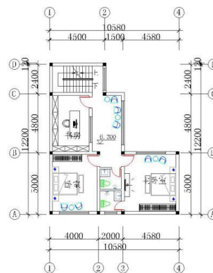
三层平面布置图 1:200
