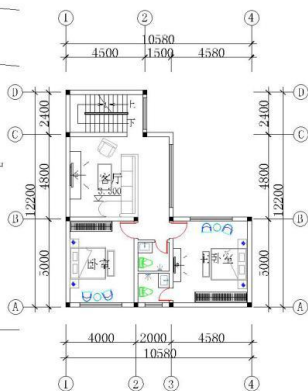
二层平面布置图 1:200
