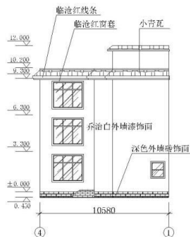
④—①轴立面图 1:200
