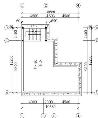
四层平面布置图 1:200
