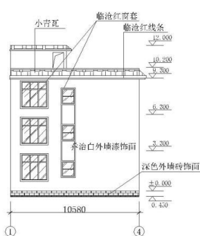
①—④轴立面图 1:200
