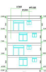
背立面图 1:100
