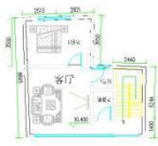
四层平面图 1:100 本层建筑面积:166.15m²
