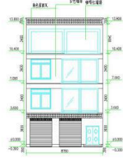
正立面图 1:100
