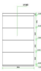
右立面图 1:100
