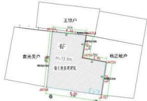
总平面布置图 1:100
