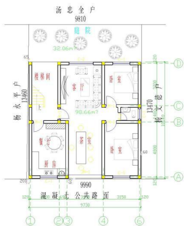
一层平面图 1:100
