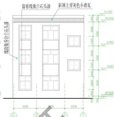
背立面图 1:100
