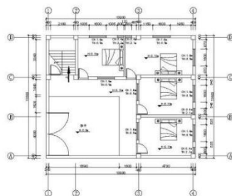
一层平面布置图 (注:一层层高:4m) 1:75 一层建筑面积:98.15m 2
