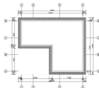
屋顶平面布置图 (注:屋顶层高:4m) 1:75 屋顶面积:147.28㎡
