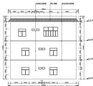
④-① 建筑左立面图 占地面积: 188.67m 2 1:75
