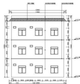
④-① 建筑背立面图 占地面积: 186.67m 2 1:75
