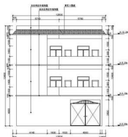
①-④ 建筑正立面图 占地面积: 186.67m 2 1:75
