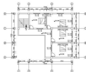
二层平面布置图 (注: 二层层高: 4m) 1:75 二层建筑面积: 98.15m 2
