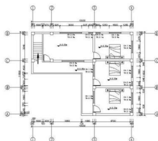
三层平面布置图 (注:三层层高:4m) 1:75 三层建筑面积:98.15m 2
