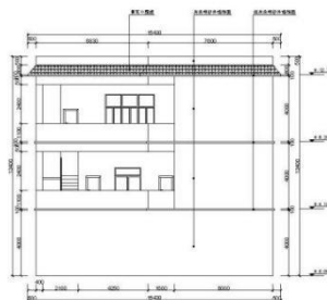
①-④ 建筑右立面图 占地面积: 186.67m 2 1:75
