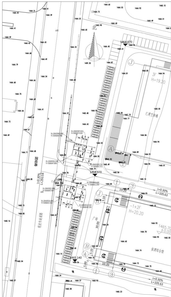
总平面布置图 1:500
